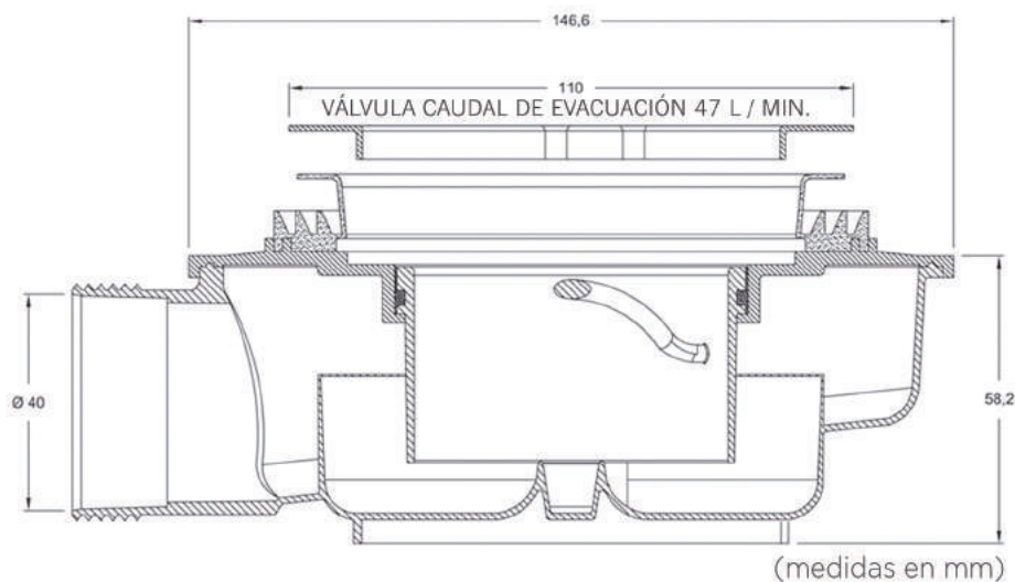
VÁLVULA SIFÓNICA EXTRA PLANA
