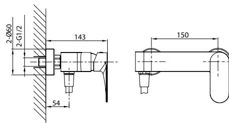
Válvula redonda ref. 0351
